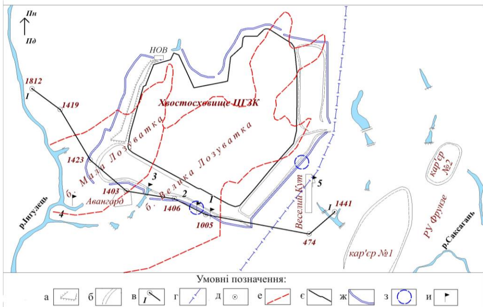
Рис. 1 – Карта-схема району досліджень: а – дамба хвостосховища ПРАТ «ЦГЗК»; б – контури упорних призм; в – лінія геологічного розрізу I-I (рис. 2); г – лінія водорозділу; д – гідроспостережні свердловини; е – контури балок; є – контур хвостосховища; ж – дренажна система хвостосховища; з – місця виходу джерел високомінералізованої води; и – місця відбору проб, 1-5 – номери проб
