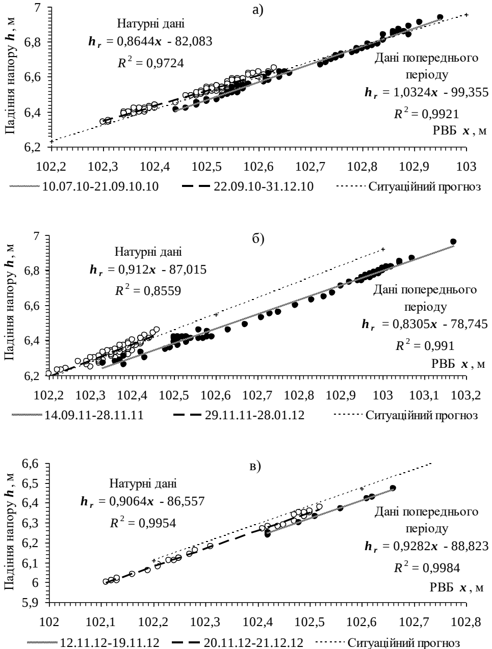
Рис. 5 – Співставлення результатів прогнозування падіння напору на ділянці фільтрації до п'єзометра П-65Б з даними спостережень в 2010 р. (а), 2011 р. (б) і 2012 р. (в)
