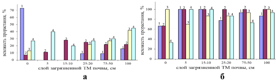
Рис. 3 – Зависимость всхожести прорастания семян салата (а) и овса (б) от слоя загрязненной ТМ почвы: 1 – дерново-оподзоленная связнопесчаная, 2 – луговая аллювиальная супесчаная, 3 – лугово-черноземная легкосуглинистая, 4 – чернозем типичный среднесмытый тяжелосуглинистый
