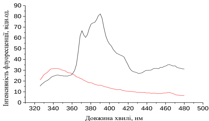
Рис. 2. – Спектри флуоресценції мембранних препаратів у відсутності (1) або присутності (2) 5 мкМ пірену, \lambda_{\text{зб}} = 280 \text{ нм}
