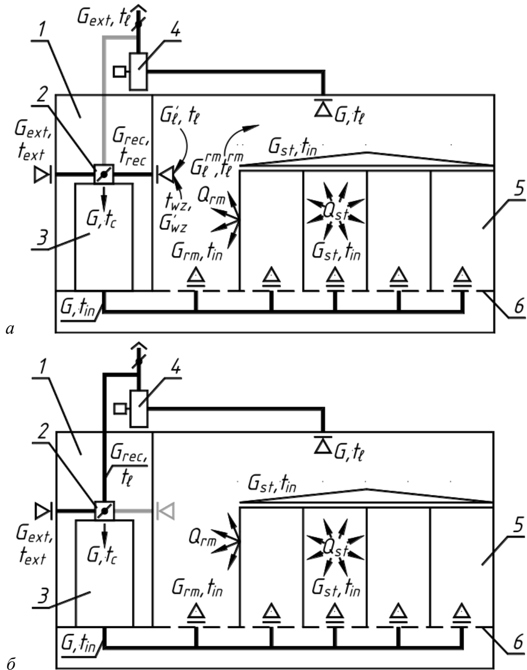
Рис. 2. Схема організації повітрообміну в дата-центрах: а – у теплий період року; б – у холодний період року: 1 – приміщення; 2 – клапан багатোধодовий; 3 – кондиціонер прецизійний шафовий; 4 – рециркуляційно-витяжний вентилятор; 5 – стативи; 6 – фальшпідлога; сірим виділено повітроводи, що не працюють у цей період року
