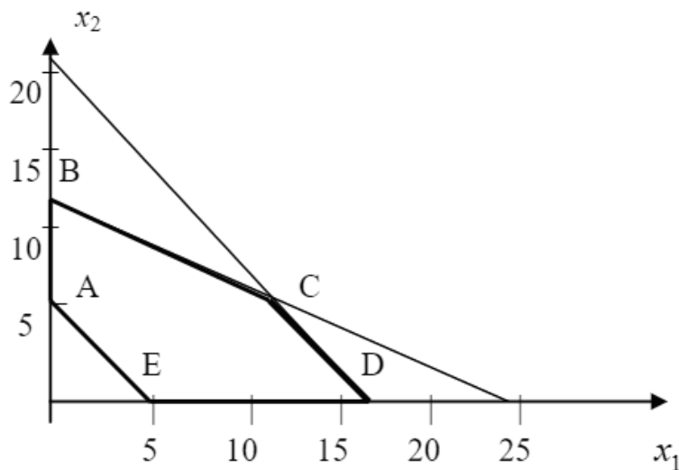
Рис. 5.2.1. Область допустимих значень
