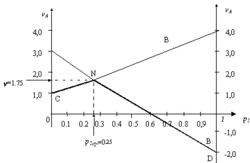
Рис. 11.3. Графічний розв'язок з позиції гравця A
