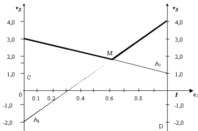
Рис. 11.4. Графічний розв'язок з позиції гравця B
