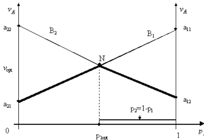
Рис. 11.1 Графічне представлення системи рівнянь 11.6
