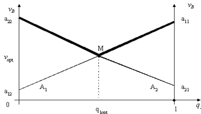
Рис. 11.2. Графічне представлення системи 11.9
