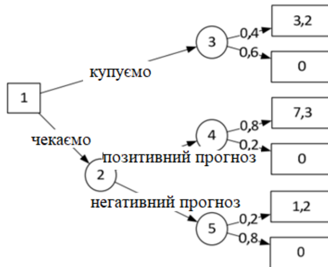
Рис 9.2. «Дерево рішень»
