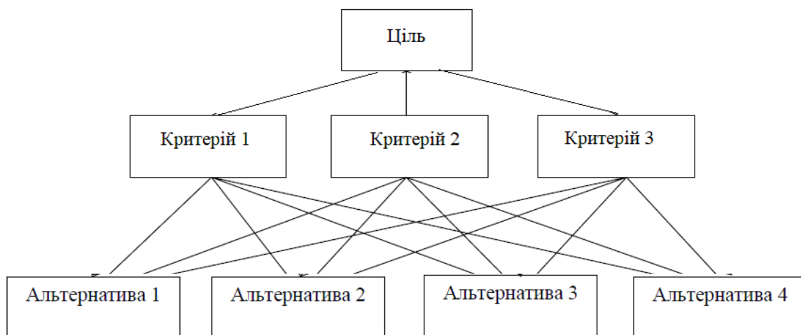
Рис. 6.1. «Дерево ієрархій»
