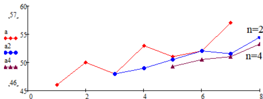
Рис. 10.1. Графіки прогнозу методом ковзного середнього
