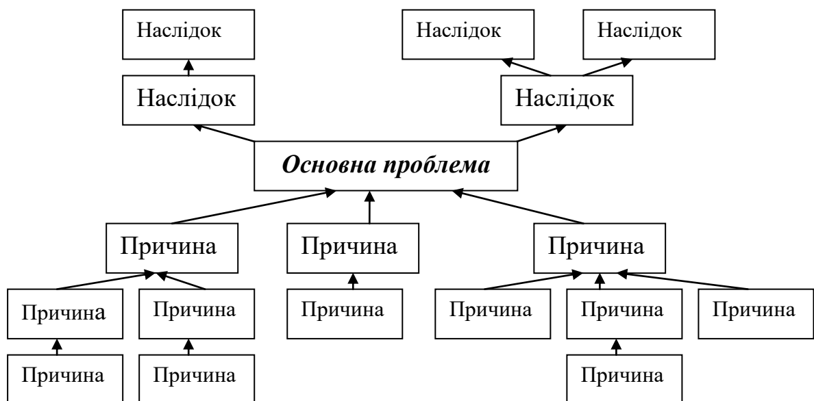
Рис. 2.1. «Дерево проблем»
