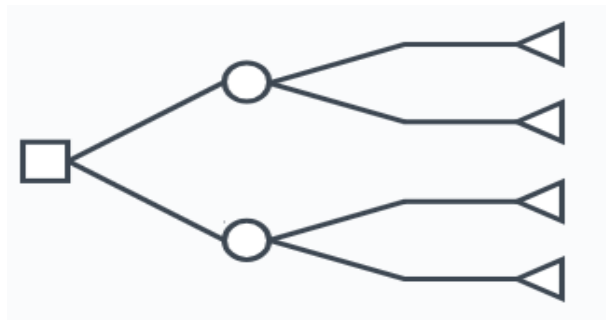
Рис. 9.1. Загальний вигляд «дерева рішень»
