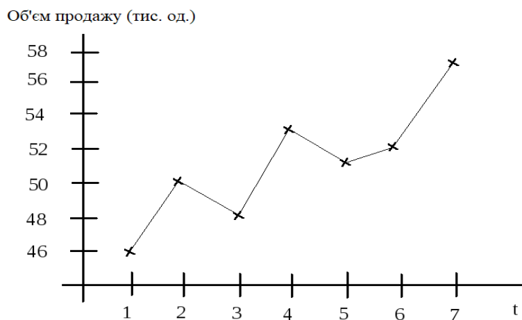
Рис. 10.2. Графік часового ряду
