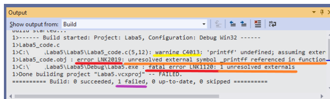
Рис. 14. Помилки під час побудови програми
