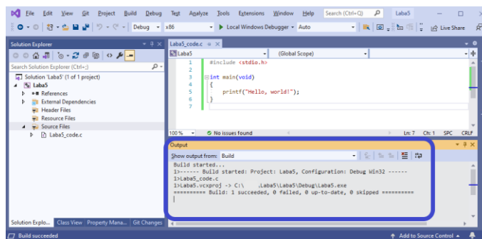
Рис. 13. Вікно Output
