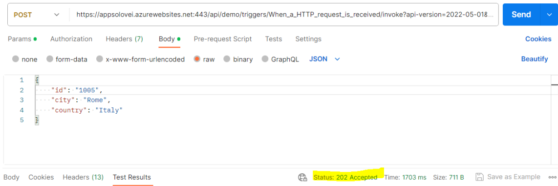
Рис. 5. 2. Приклад для визначення методу POST в Postman Web
