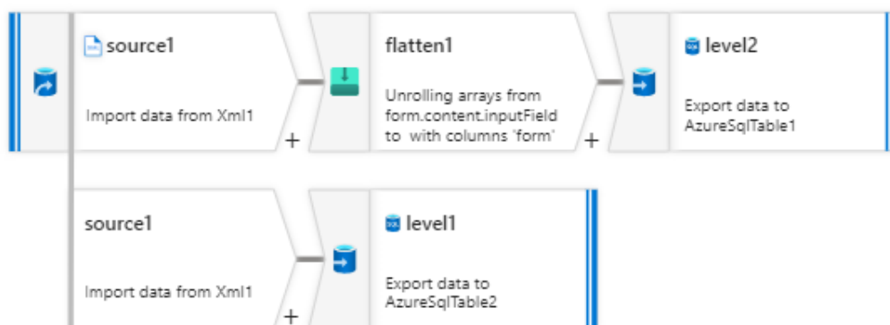
Рис. 1. Схема потоку даних для реалізації процесу ETL
