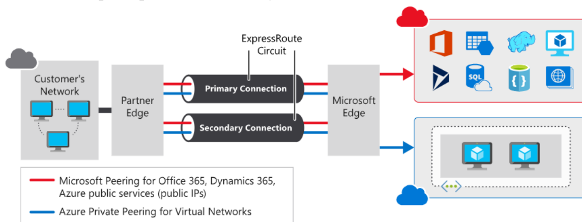
Рис. 3. 1. Архітектура з'єднання каналом ExpressRoute
