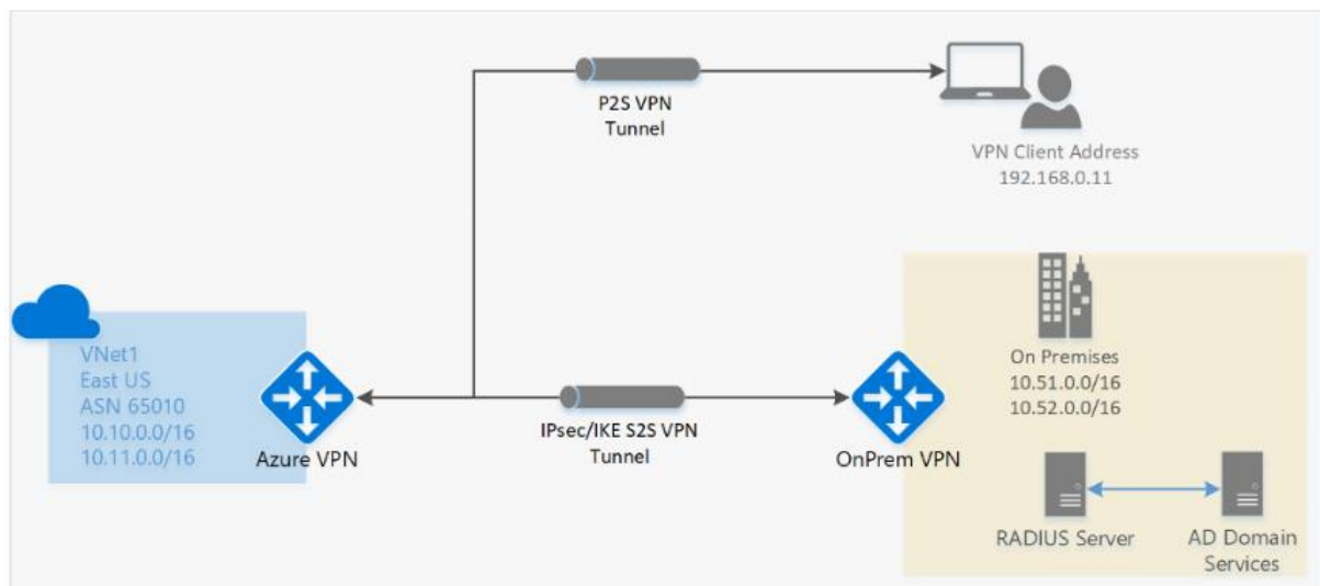
Рис. 2. 1. Конфігурація з'єднання типу «точка – мережа»
