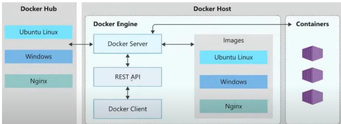
Рис. 4. 1. Архітектура контейнеру Docker в хмарному середовищі Azure
