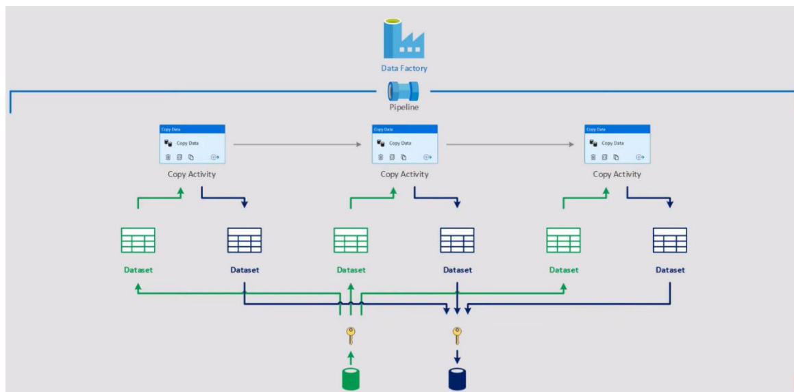
Рис. 7. 1. Конвеєр який об'єднує послідовні дії копіювання даних
