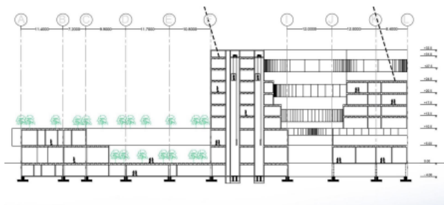
Розріз А-Л
