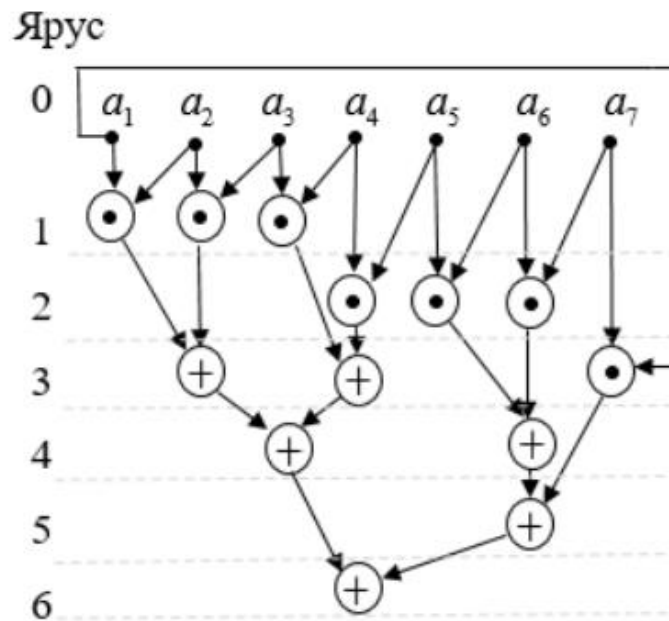
Рис. 3.2. Граф алгоритму у послідовній системі з трьома процесорами
