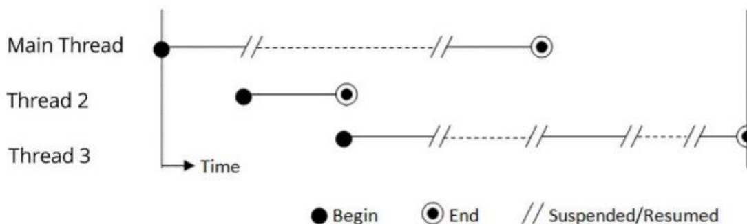
Рис. 4.1. Багатопотокова програма
