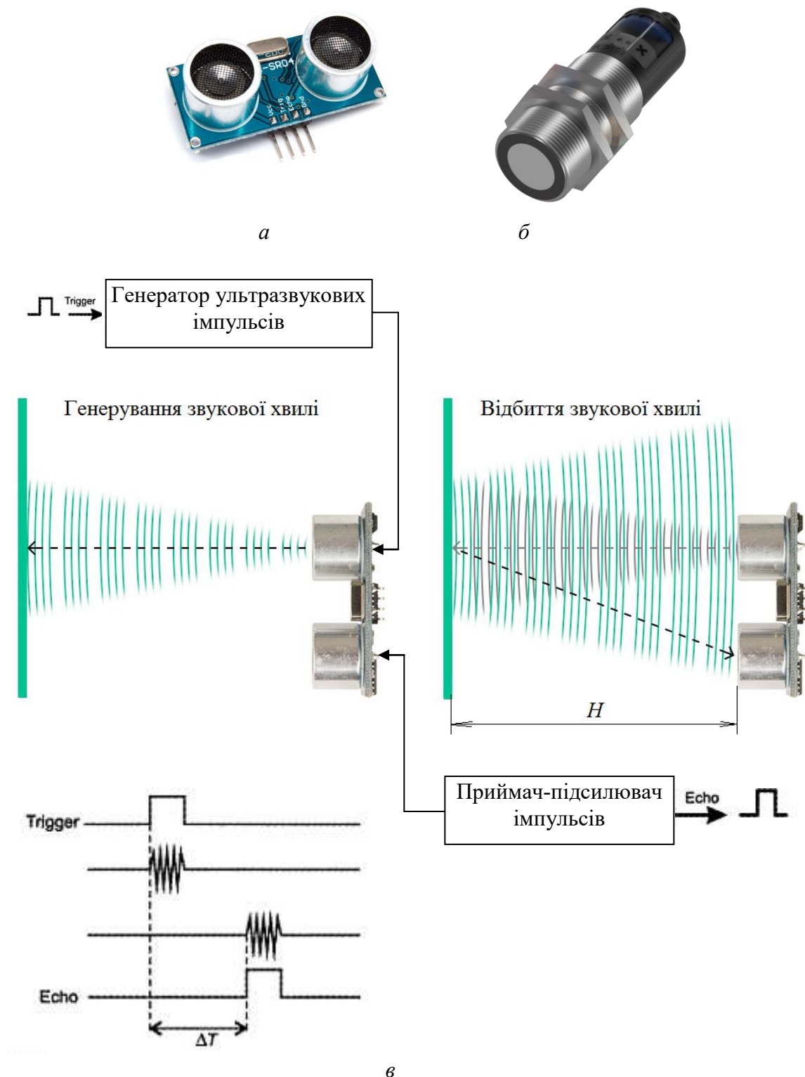
Рис. 4.5. Ультразвуковий сонар: a – модуль HC-SR04 ультразвукового сонара; б – промисловий ультразвуковий датчик BUS003F; в – принцип роботи сонара
