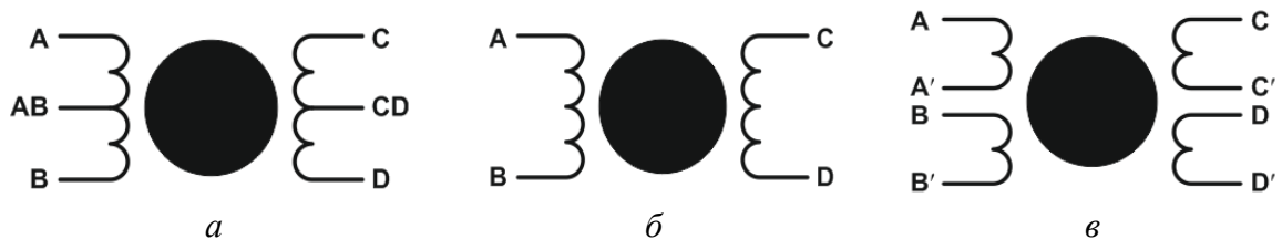
Рис. 5.8. Схеми ввімкнення обмоток статора крокових двигунів: а – уніполярна; б – біполярна; в – з роздільним виводом обмоток
