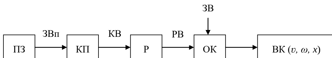
Рис. 9.1. Процеси системи керування: ПЗ – програмний задатчик; КП – керівний пристрій; Р – регулювальний орган; ОК – об'єкт керування; ВК – вихідні координати; ЗВп – заданий вплив; КВ – керівний вплив; РВ – регулювальний вплив; ЗВ – збурювальний вплив
