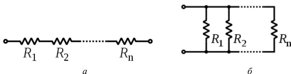
Рис. 4.2. Схеми послідовного (а) та паралельного з'єднання провідників (б)
