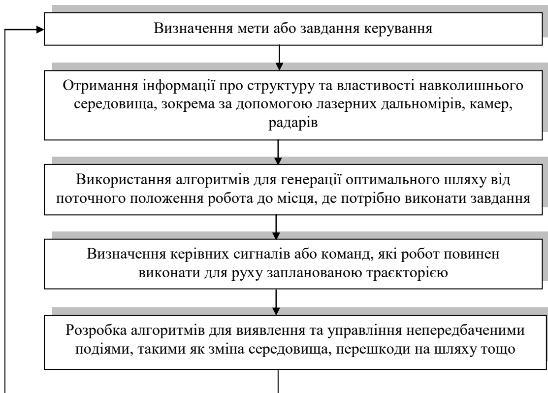
Рис. 7.11. Алгоритм керування на основі добору траєкторії
