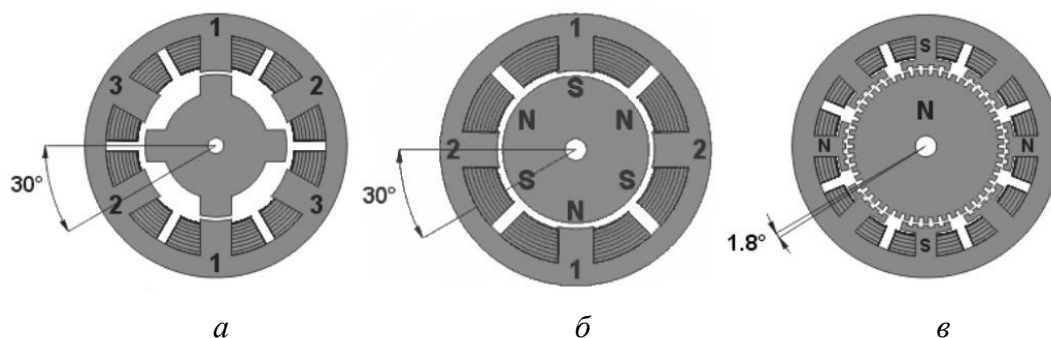
Рис. 5.7. Конструкції крокових двигунів: а – зі змінними магнітами; б – з постійними магнітами; в – гібридний
