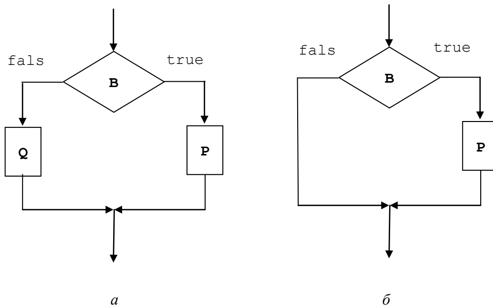
Рис. 7.7. Алгоритм з повним (а) та неповним (б) розгалуженням
