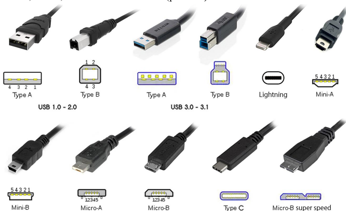
Рис. 8.2. Різновиди типів USB
