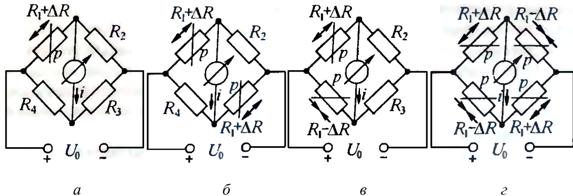
Рис. 4.18. Схеми вмикання тензорезисторів: а – мостова схема з одним тензорезистором; б та в – мостові схеми з компенсацією температурної похибки; г – мостова схема ввімкнення тензодатчиків підвищеної чутливості (міст Вітстона) (тензорезистори на схемі зображено у вигляді змінних резисторів)
