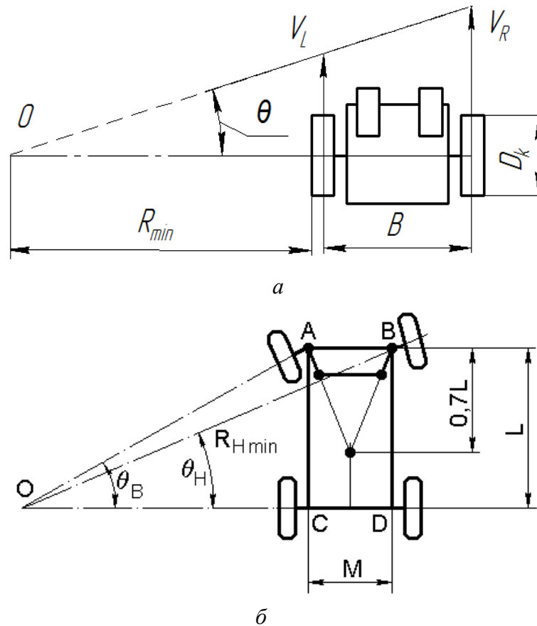
Рис. 3.2. Схеми транспортних робіт: а – з бортовим поворотом; б – з маневреними колесами: В, М – колія; L – база; R_{\min} – радіус повороту; V_L , V_R – швидкість лівого та правого коліс відповідно
