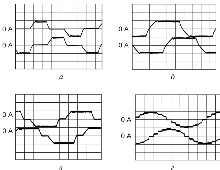
Рис. 5.9. Діаграми зміни струму в обмотках біполярного крокового двигуна для різних режимів керування: а – хвильовий; б – повнокроковий; в – напівкроковий; г – мікрокроковий
