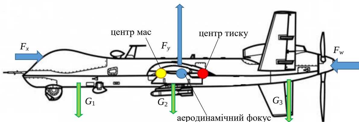
Рис. 2.12. Схема центрування БПЛА з жорстким крилом: F_y – аеродинамічна підймальна сила; F_x – сила аеродинамічного опору; F_w – сила тяги; G_1 – сила ваги обладнання; G_2 – сила ваги корпусу; G_3 – сила ваги силової установки
