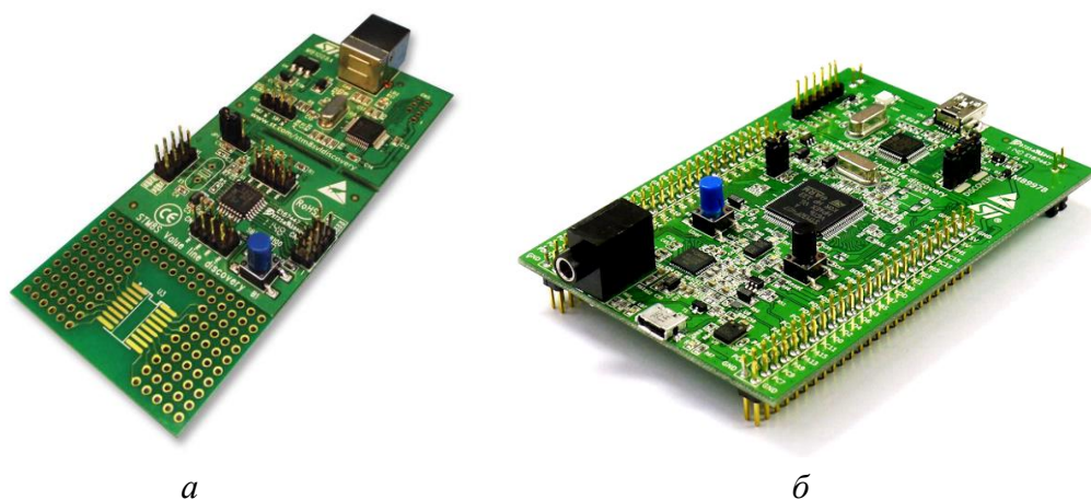
Рис. 5.26. STM мікроконтролери: а – STM8S-Discovery; б – STM32VL-Discovery
