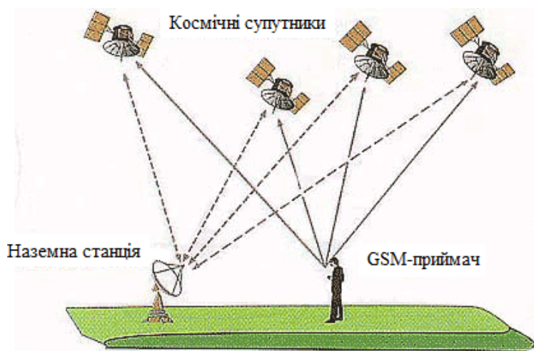
Рис. 5.16. Принцип роботи системи GPS
