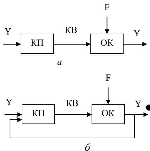
Рис. 9.2. Різновиди систем керування: а – розімкнена; б – зі зворотним зв’язком; КП – керівний пристрій; КВ – керівний вплив; F – перешкоди; X – вплив, що задається; Y – вихідні координати
