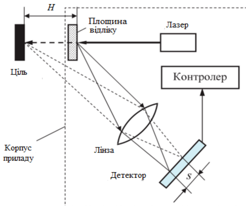
Рис. 4.10. Принцип роботи оптичної лазерної тріангуляції
