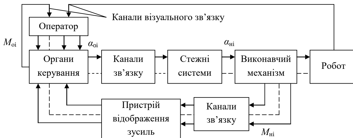
Рис. 9.6. Блок-схема оберненої стежної системи
