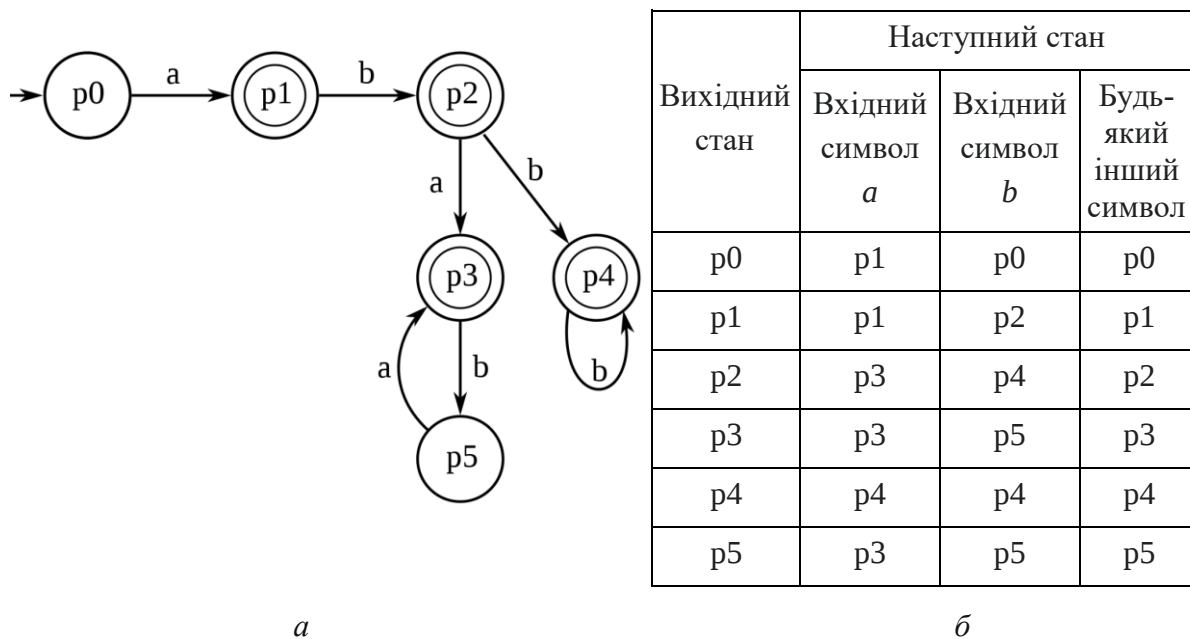
Рис. 8.19. Способи представлення скінченних множин станів: a – приклад детермінованої системи; б – у вигляді таблиці
