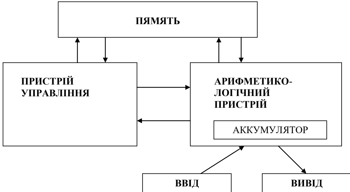
Рис. 5.21. Архітектура Фон-Неймана
