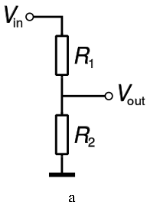
Рис. 4.13. Схема ділильника напруги (а) та вигляд змінного резистора (потенціометра) (б)
