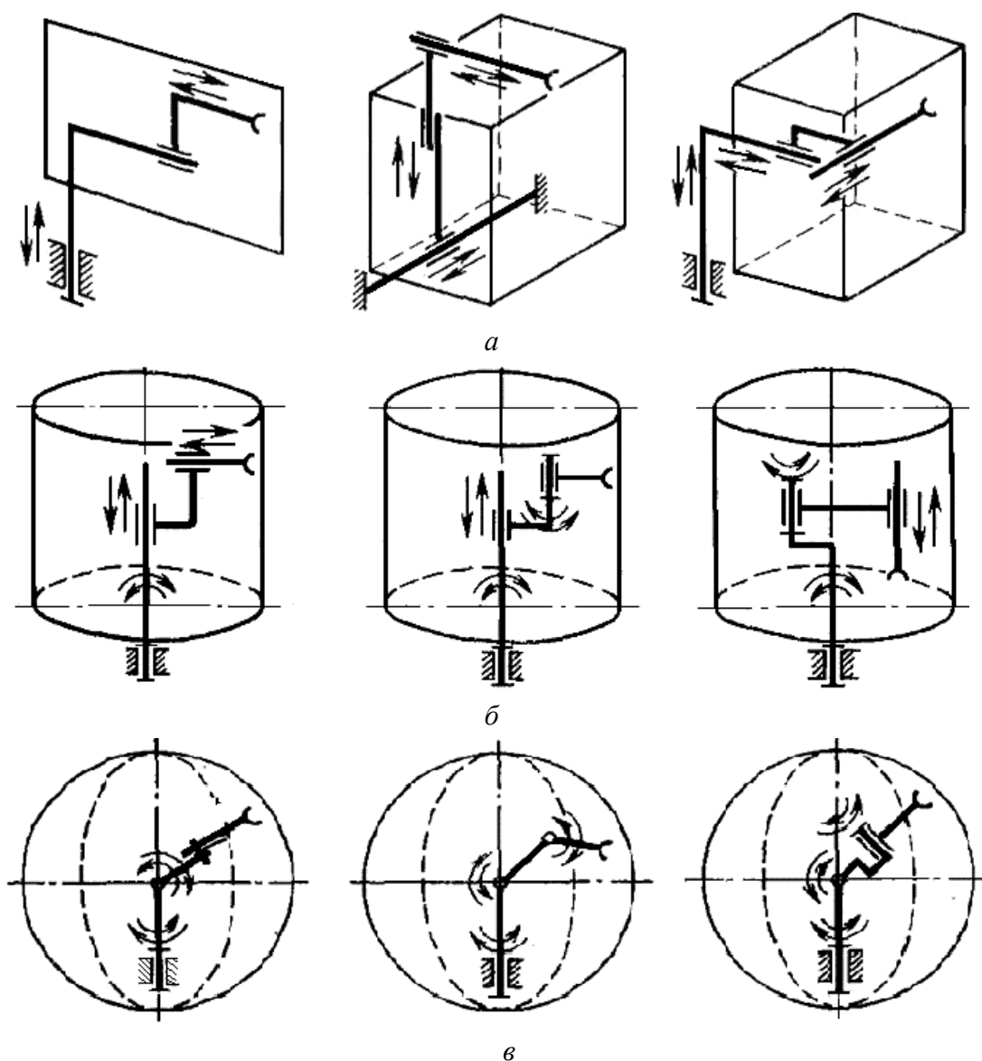
Рис. 1.7. Структурні схеми роботів: а – прямокутна система координат; б – полярна циліндрична система координат; в – полярна сферична (ангулярна) система координат
