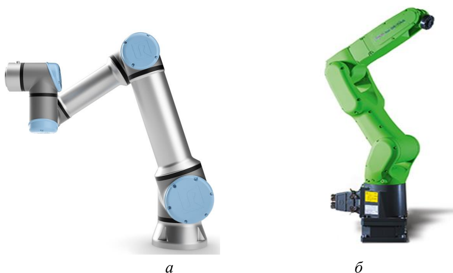
Рис. 1.6. Колоборативні роботи-маніпулятори UR16e (Universal Robots) ( а ) та CR-7iA/L (Fanuc) ( б )
