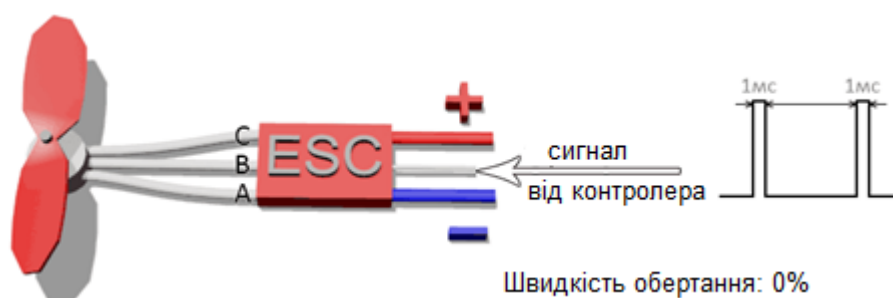
Рис. 2.14. Схема під'єднання ESC до електродвигуна
