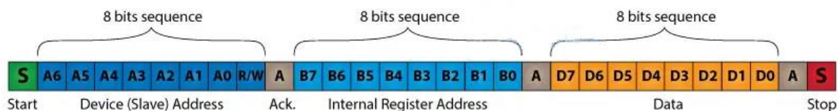
Рис. 8.6. Вигляд протоколу транзакції даних I2C: Device (Slave) Address – адреса пристрою, який приймає дані; Ack – підтвердження від пристрою, що приймає; Internal Register Address – адреса внутрішнього реєстру; Data – дані
