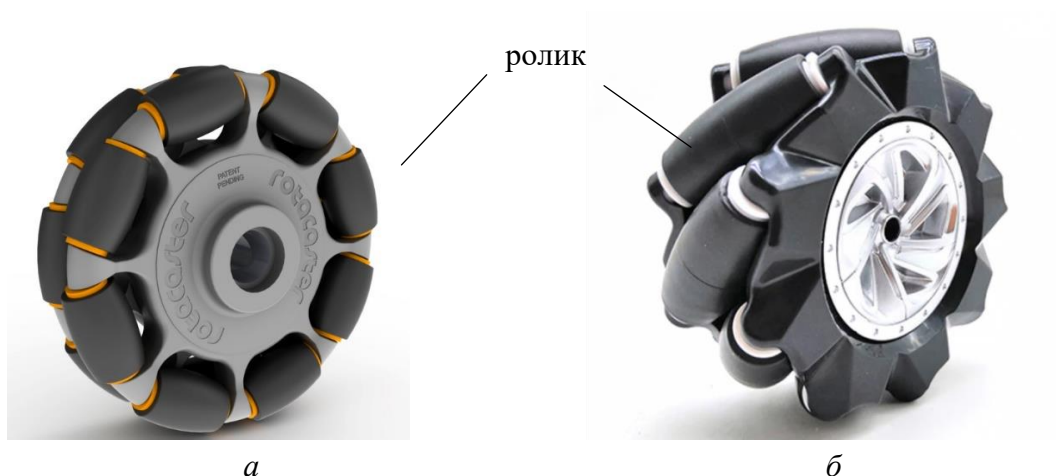
Рис. 1.12. Вигляд омні-колеса ( a ) та колеса Ілона (меканум-колесо) ( б )
