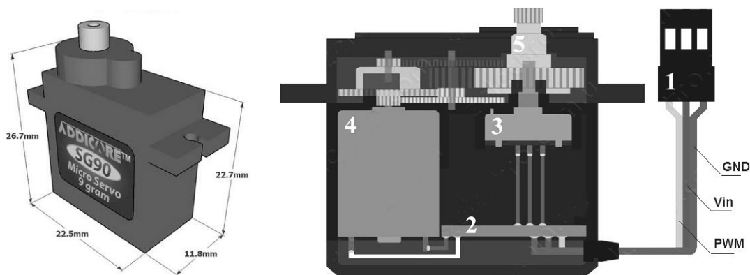
Рис. 5.3. Конструкція лабораторного сервоприводу: 1 – комутаційний рознімач; 2 – внутрішня плата керування; 3 – потенціометр; 4 – колекторний електродвигун; 5 – вихідний вал редуктора; Vin – вхід живлення; GND – «земля»; PWM – сигнал керування
