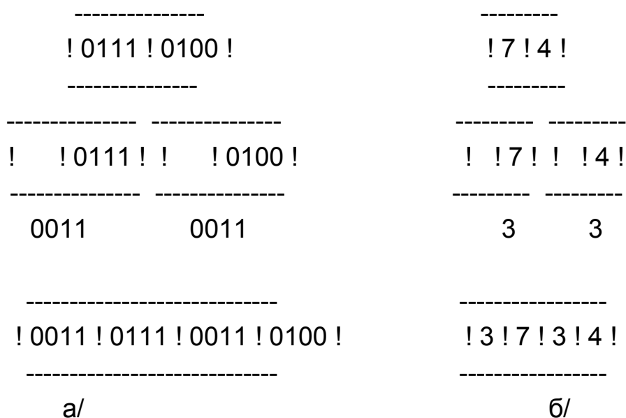
Рис. 1.1. Формування ASCII-кодів для десяткового числа 74
