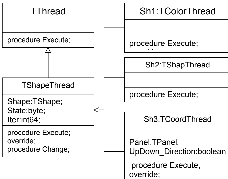
Рис. 5.1. Ієрархія класів потоків
