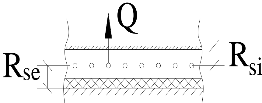
Рис. 5. Опори теплопередачі підлоги
