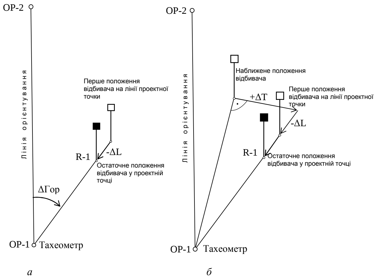
Рис. 2.2. Розмічування проектної точки: а – перший варіант; б – другий варіант
