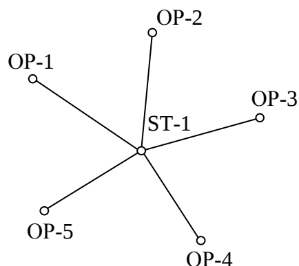
Рис. 3.1. Зворотна засічка
