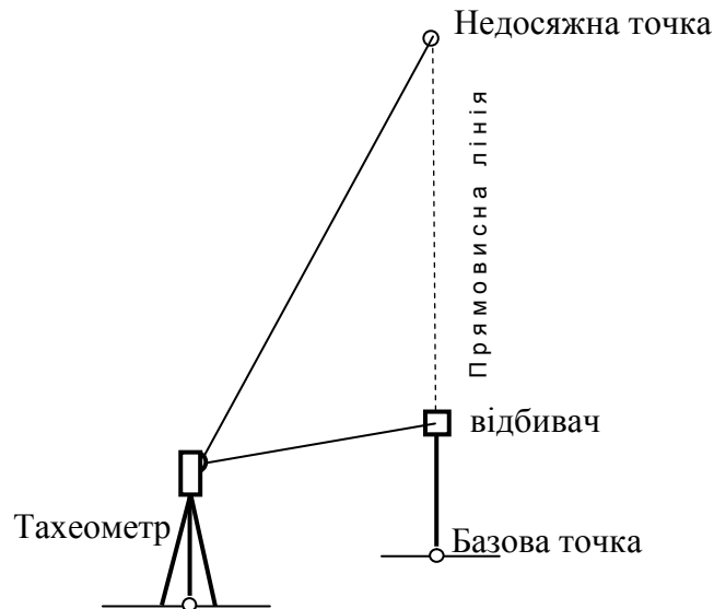
Рис. 7.1. Визначення висоти недоступної точки
