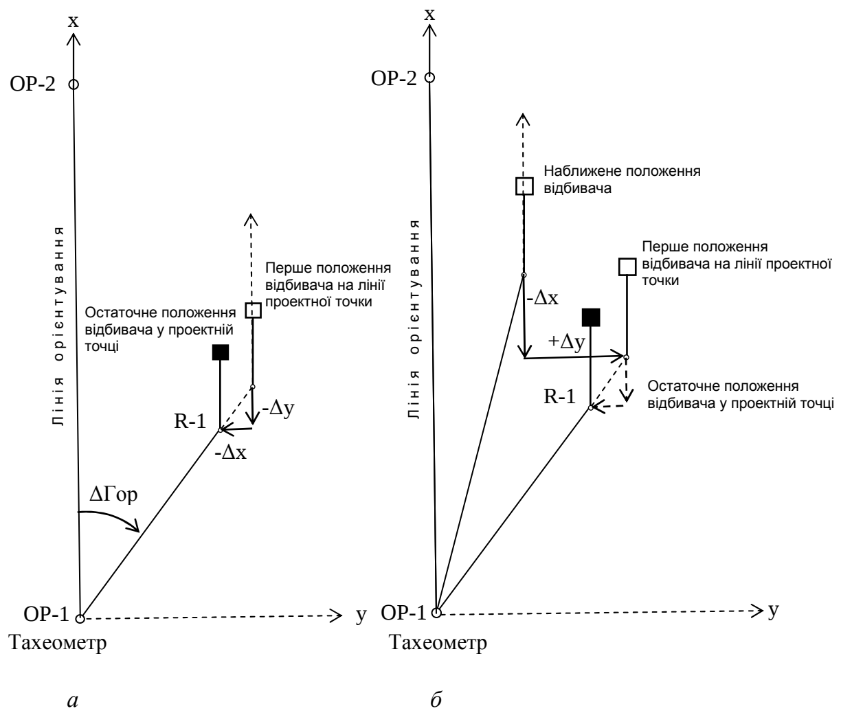
Рис. 2.3 Розмічування проектної точки: а – перший варіант; б – другий варіант
