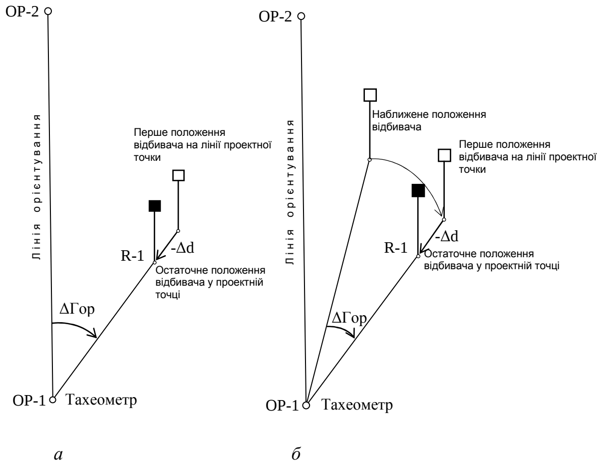
Рис. 2.1. Розмічування точки: а – перший варіант; б – другий варіант
