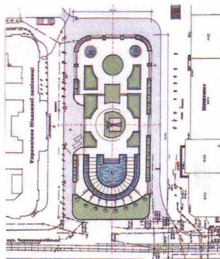
Рис. 9. Генсхема Привокзальної площі в м. Харкові
