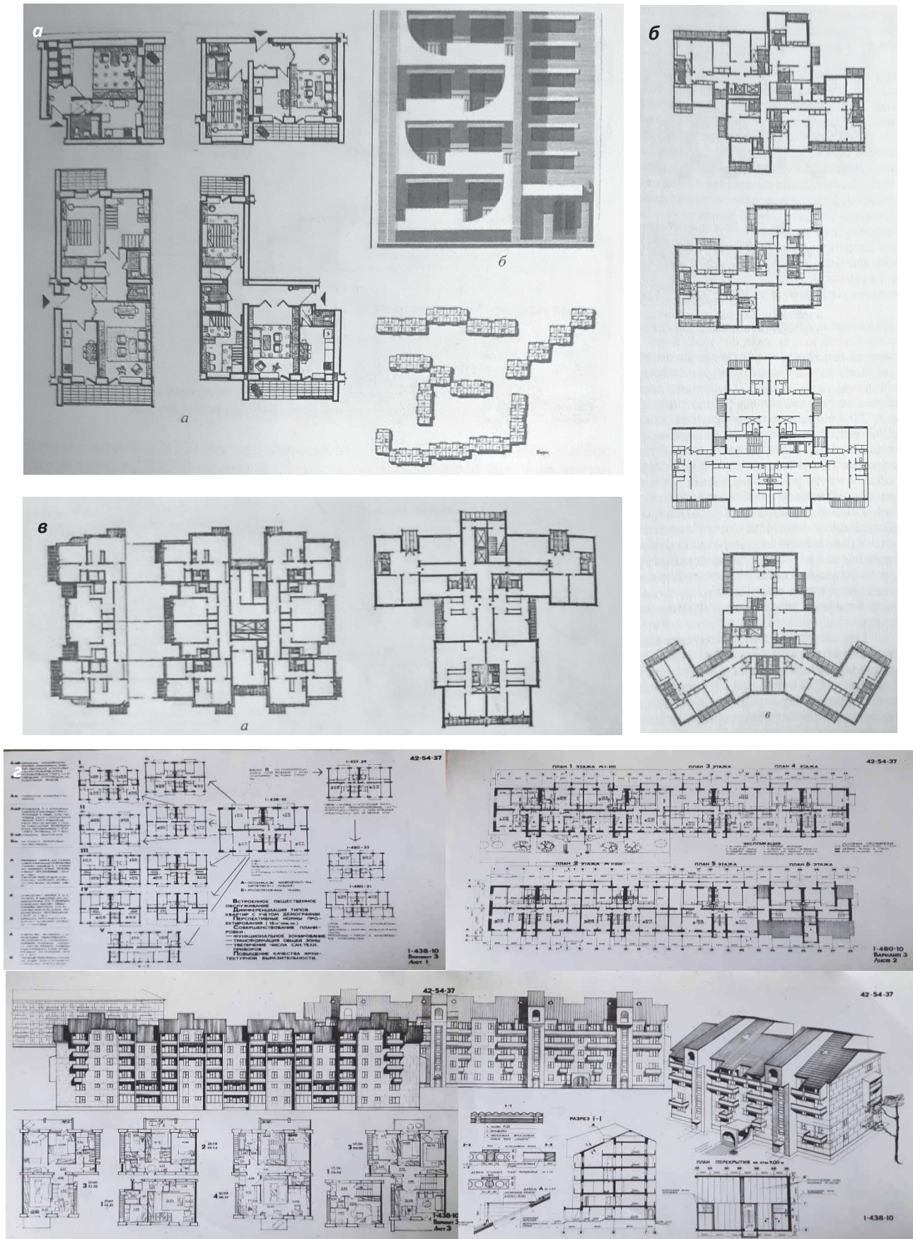
Рис. 2. Проекти: а – Серія типових 5-пов. будинків для буд-ва у сейсмічних р-нах Криму і Карпат, КиївЗНДІЕП, 1976; б – Проект нових типів житл. будинків для масового буд-ва, КиївЗНДІЕП, 1978; в – Проект перспективних типів житл. будинків для масового буд-ва, Київпроект, 1978; г – конкурсний проект реконструкції 5-пов. будинків, 1986.
